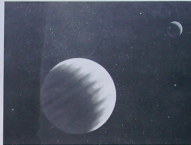
Ίσως ο δορυφόρος Τρίτων να άσκει τέτοια επίδραση στο δακτύλιο του Ποσειδώνα, ώστε ο πλανήτης αυτός να άποτελεί μία ιδιόμορφη εξαίρεση στο ήλιακό μας σύστημα.
