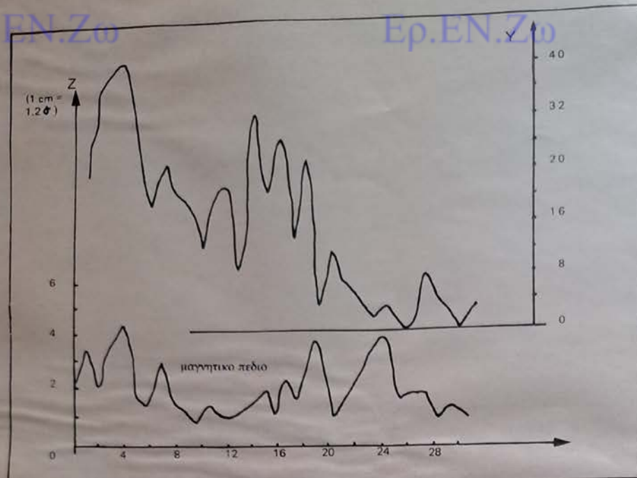
Είκ. 4. Διαγράμματα για τη σύγκριση της κατανομής των εμφανίσεων UFO με την κατανομή των διαταραχών στην κάθετη συνιστώσα του γήινου μαγνητικού πεδίου. CHAMBON-LA-FORET. Οκτώβρης 1954.
