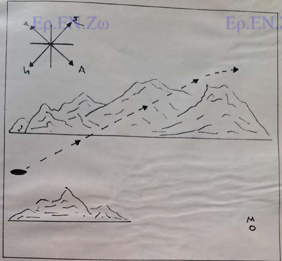
Σχ. 3. Τά UFO πέρασαν με μεγάλη ταχύτητα πάνω από κάτι κοντινούς λόφους και πλησιάζοντας τα βουνά χάθηκαν πίσω απ'αυτά (πάνω).
