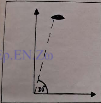
Σχ.1 και Σχ. 4. Τη στιγμή της εμφάνισής τους σχημάτιζαν μία γωνία 80 μοιρών περίπου με το επίπεδο εδάφους των παρατηρητών (πάνω και κάτω).
