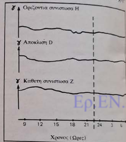
Είκ 1. Τυπική καταγραφή τού γήινου μαγνητικού πεδίου στη διάρκεια εμφα- νίσης UFO. 'Η κάθετη διακεκομμένη γραμμή παριστάνει τό χρόνο της πα- τήρησης πού έγινε από απόσταση 58 χιλιομέτρων στις 24 τού Μάη τό 1954 στις 22.15.
