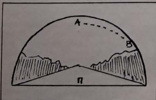
Σχ.1 και Σχ. 4. Τη στιγμή της εμφάνισής τους σχημάτιζαν μία γωνία 80 μοιρών περίπου με το επίπεδο εδάφους των παρατηρητών (πάνω και κάτω).
