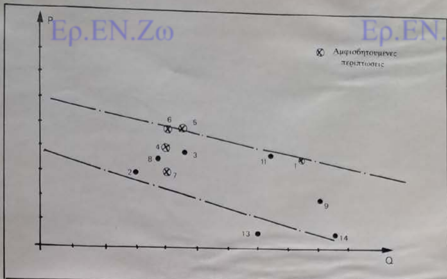
Εικ. 2. Άξονας P- Διαμόρφωση των ολικών μεταβολών κατά μία χρονική διάρκεια 3 ωρών πριν και μετά από μία παρατήρηση UFO. Άξονας Q= απόσταση σε χιλιόμετρα των UFO από το CHAMBON-LA-FORET
